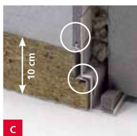
Spodní víko s dvojitým falcem, 10cm izolace a dvojitě těsnění
