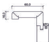
FU-RF 60/16 mm
