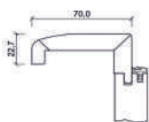
FU-SLF 70/22,7 mm
