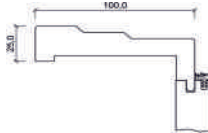
FU-PM 100/25 mm
