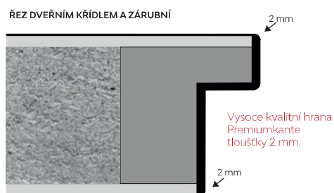
DVEŘNÍ KŘÍDLO S HRANOU PREMIUMKANTE (PK)
